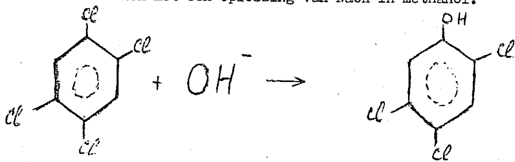
1,2,4,5-tetrachloorbenzenen
